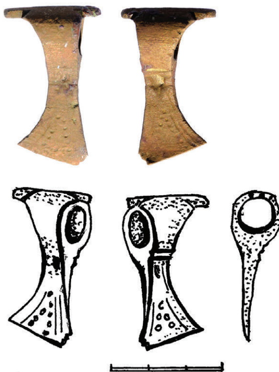
Обр. 2. Бронзова бравичка от Дръстър (Силистра) открита през 2015 г. източно от североизточния ъгъл на цитаделата на града (снимка и рисунка по Г. Атанасов)
