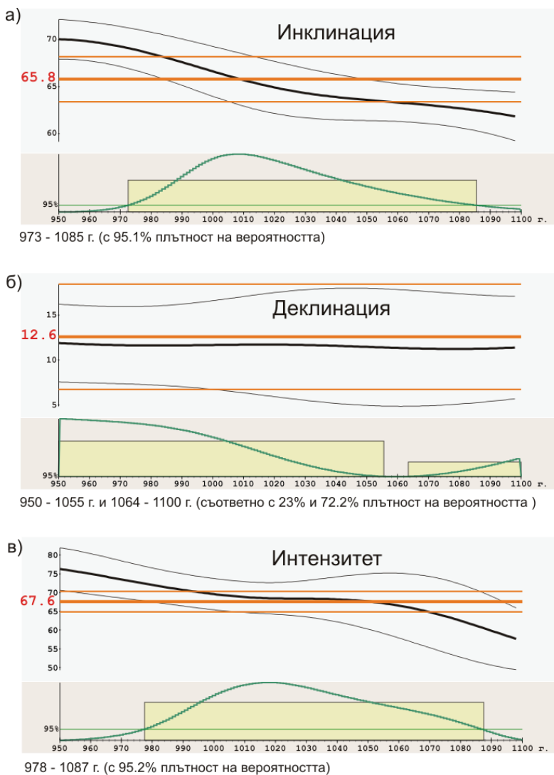
Обр. 4. Съпоставяне на получените археомагнитни резултати със съответните реперни криви за България: а) инклинация; б) деклинация; в) интензитет
