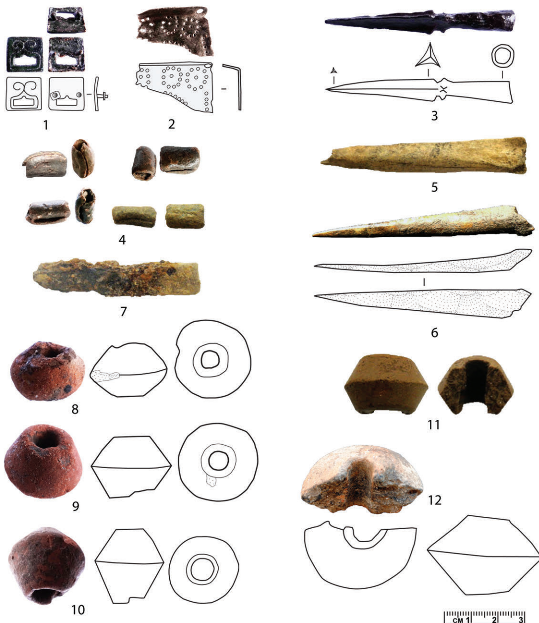
Обр. 8. Находки от средновековния културен пласт на обект № 5: 1. Бронзова апликация; 2. Сребърна пластина; 3. Врх на стрела; 4. Оловни тежести за рибарски мрежи; 5-6. Костени шила; 7. Нож; 8-12. Прешлени за вретено
