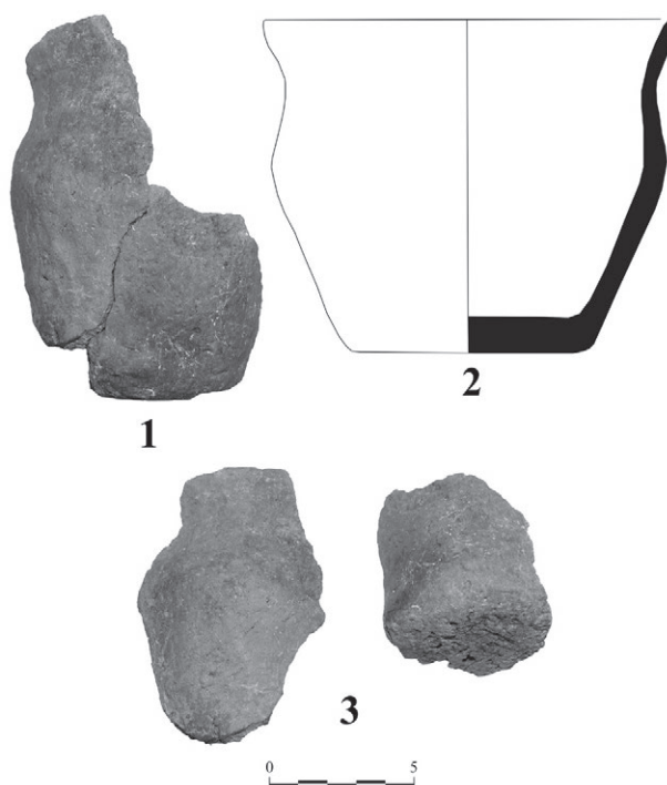
Обр. 8. Ранносредновековно гърне, изработено на ръка: 1. снимка; 2. рисунка; 3. детайли. Рисунка К. Чакъров.
