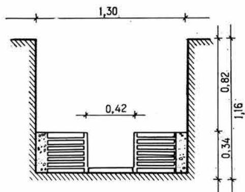
Разрез по А-А
