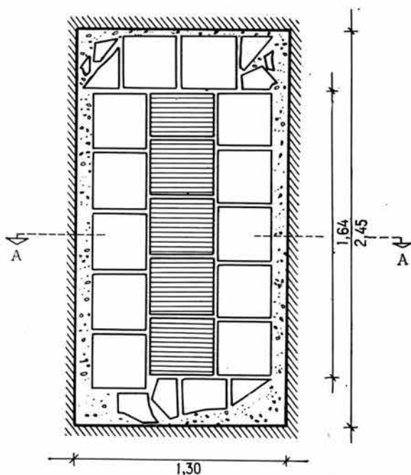
План М 1:20
