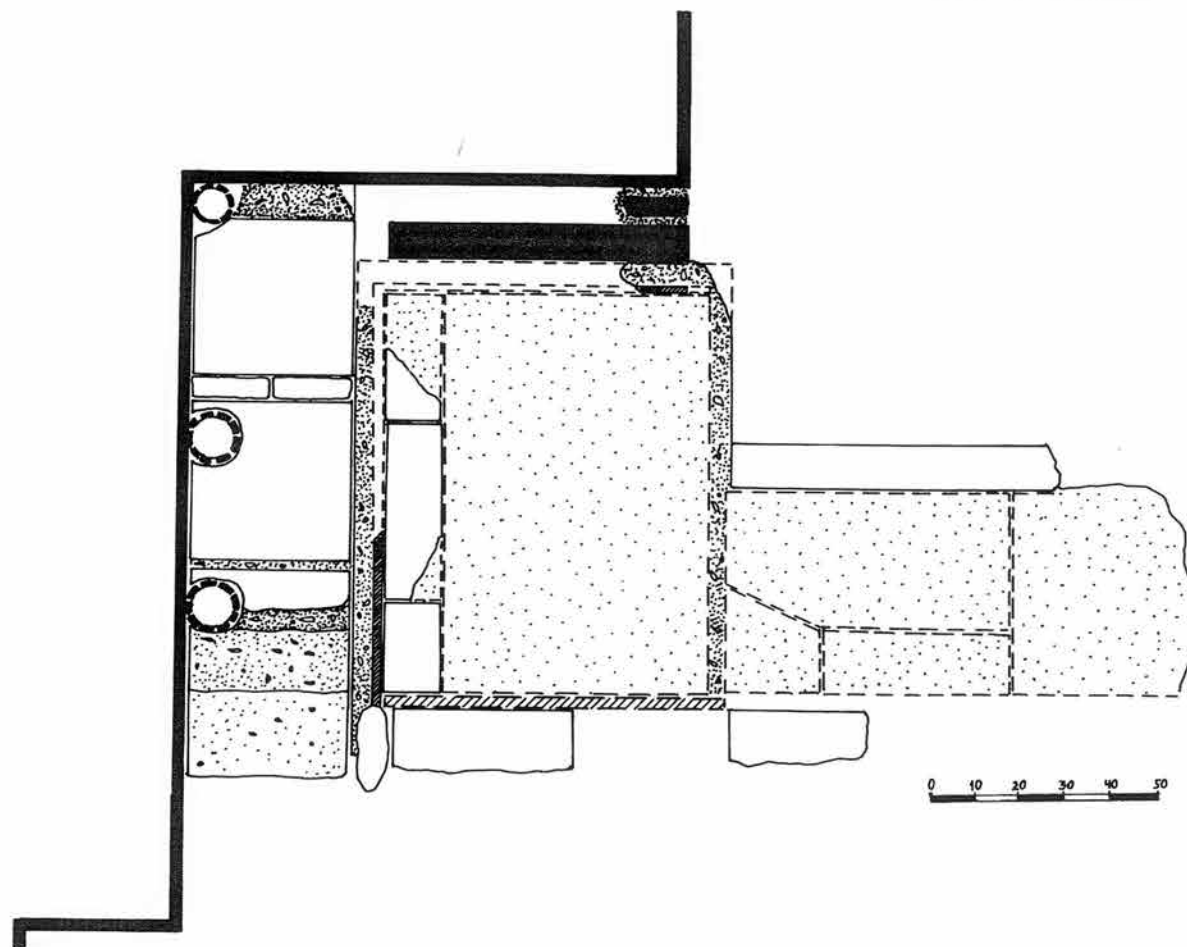
● Обр. 11. Разрез в помещение 6 (поглед от изток). Fig. 11. Coupe du local 6 (vue de l'Est)
