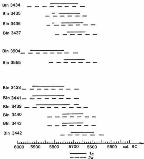
● Обр. 1. Калибрационни интервали на C-14 датите от голямата къща в Слатина. Fig. 1. Des intervalles de calibrage des dates C-14 de la grande maison à Slatina
