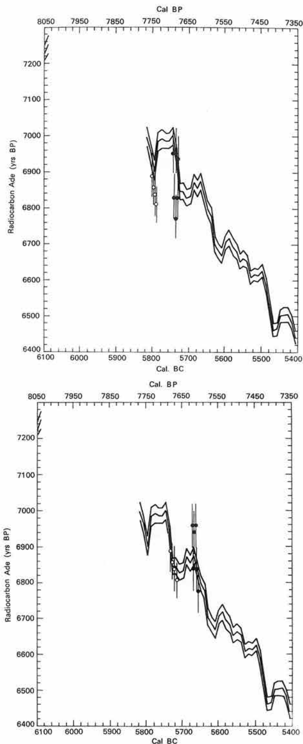
● Обр. 2. Възможно разположение на отделните групи C-14 дати върху калибрационната крива на Линик и др. Fig. 2. Une probable disposition des divers groupes de dates C-14 sur la courbe de calibration de Linnick
