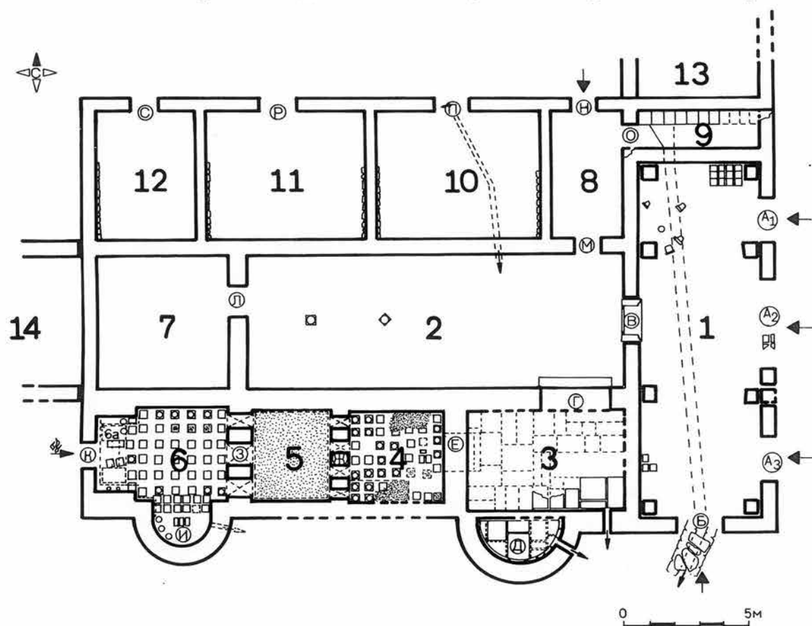
• Обр. 1. План на банята в Никополис ад Нестум. Fig. 1. Plan des bains à Nicopolis ad Nestum
