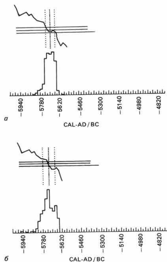
• Обр. 3. Калибрация на усреднените C-14 дати: а) за група 1а; б) за група 2. Fig. 3. Le calibrage des dates C-14 moyennes: а) du groupe 1а; б) du groupe 2
