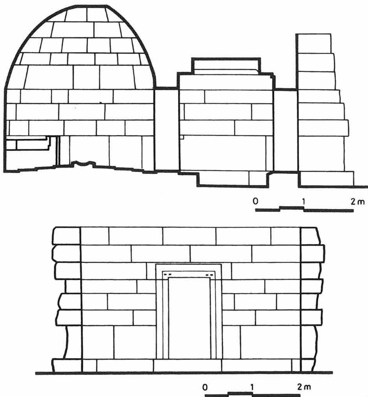
•Обр. 5. План и разрез на гробницата-мавзолей. Fig. 5. Plan et coupe de la tombe-mausolée
