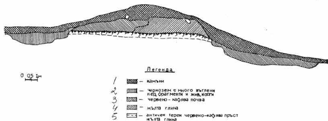
• Обр. 3. Профил на крепостната стена и рововете на сондаж I на крепостта при с. Кралево, Търговишко
