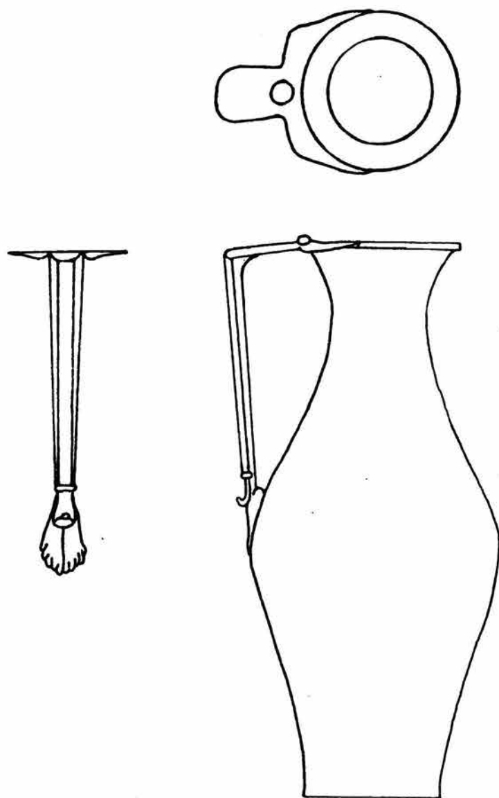
• 2. Бронзова кана от с. Садина, Поповско. М 1:3
