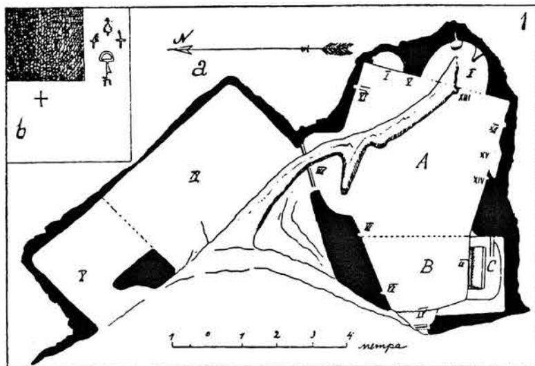
• Обр. 2. План на пещерната църква „Манастира“ (по К. Шкорпил). Fig. 2. Plan de l'église rupestre dite "Manastira" (d'après K. Škorpil).
