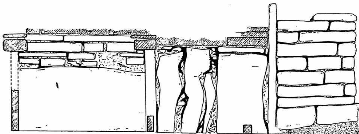
Обр. 6. Западната стена на гробницата-разрез. Fig. 6. Le mur occidental de la tombe.
