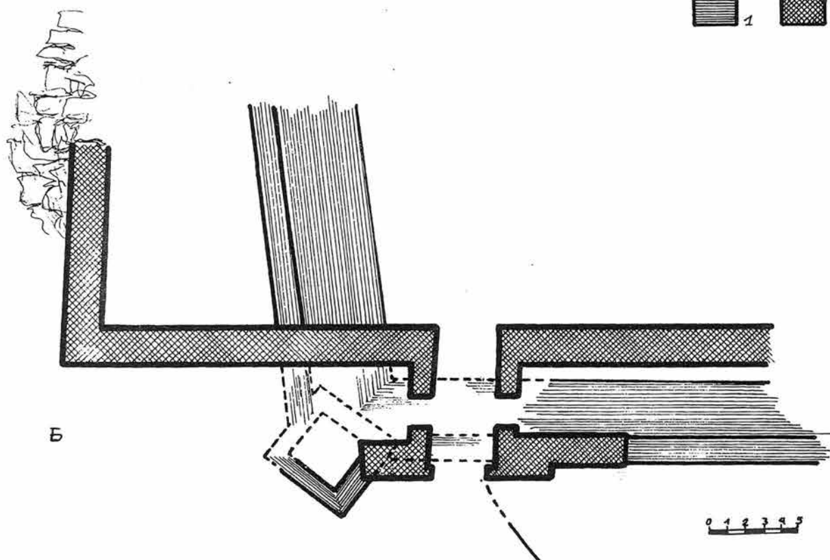
Обр. 7. а) План на вход № 1; б.) План на вход № 2. Fig. 7. a) Plan de l'entrée № 1; b) Plan de l'entrée № 2.
