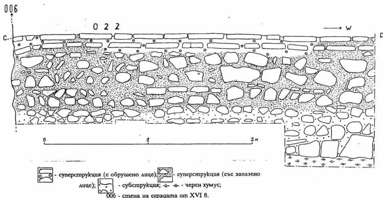
Обр. 4. Вътрешното лице на разкрития участък от южната стена (022) на сградата от края на II – първата половина на III в.
