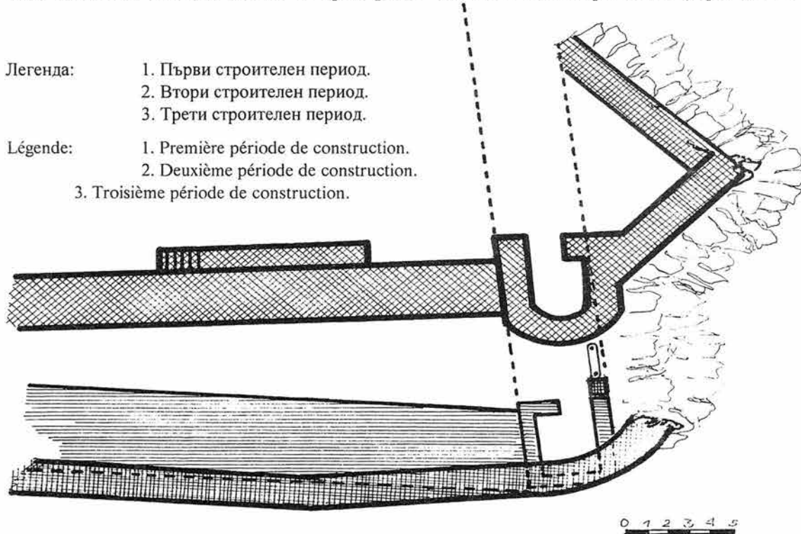
Обр. 9. Северен участък от укрепителните съоръжения – стратиграфски план.
