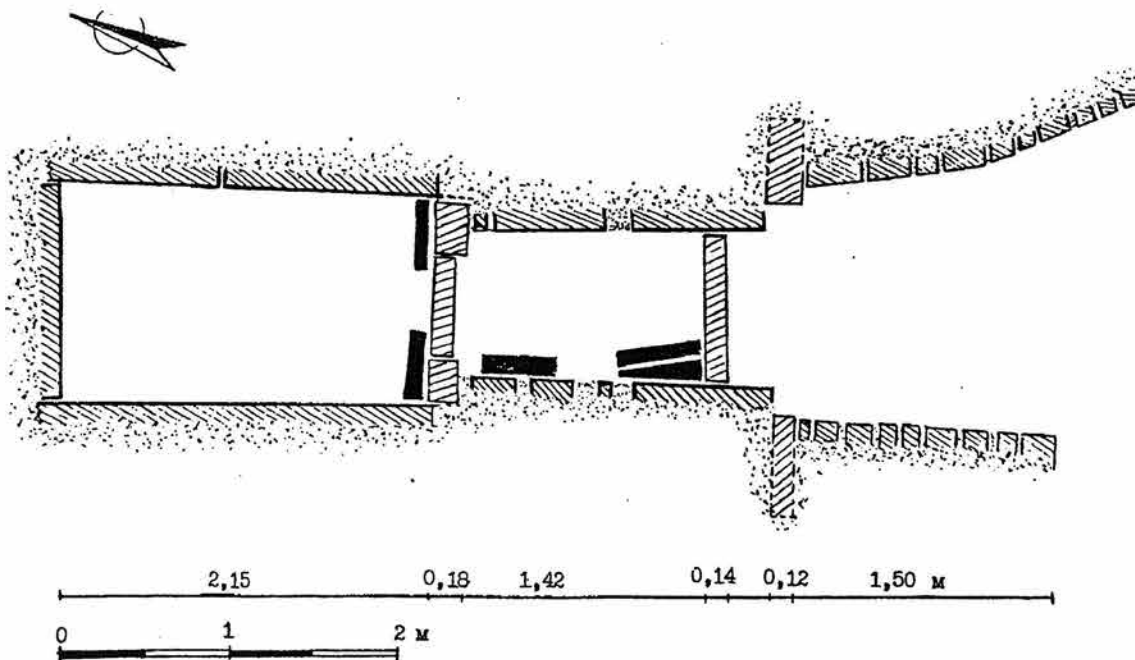
Обр. 2. План на гробницата.
