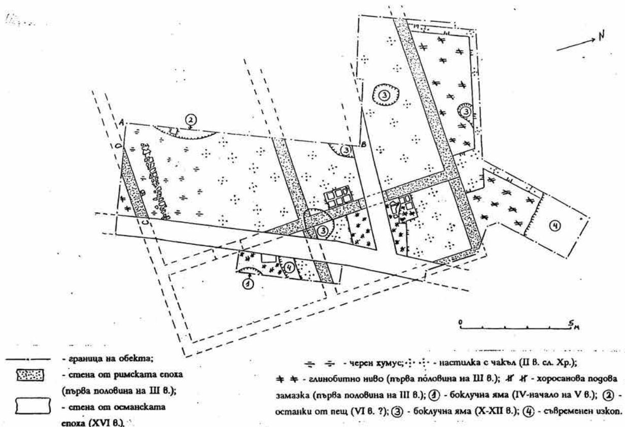
Обр. 2. План на разкритите останки (планът отразява ситуацията до нивото на настилка с чакъл от II в.). Fig. 2. Plan des vestiges mis au jour (le plan reflète la situation jusqu'au niveau du revêtement de gravier du II e s.).
