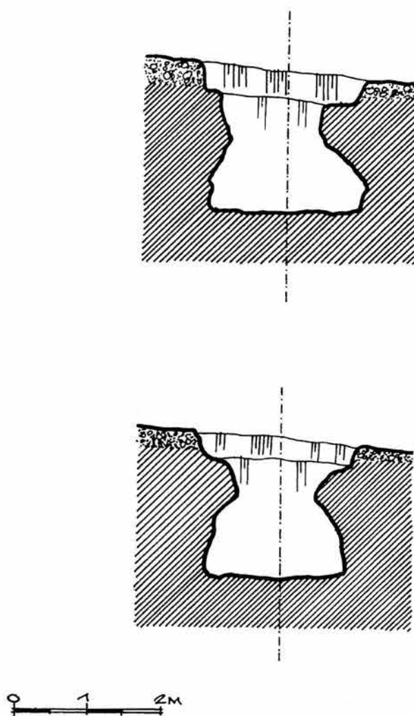
Обр. 2b. Планове и разреза на ритуални ями от местността „Костадин чешма“.
