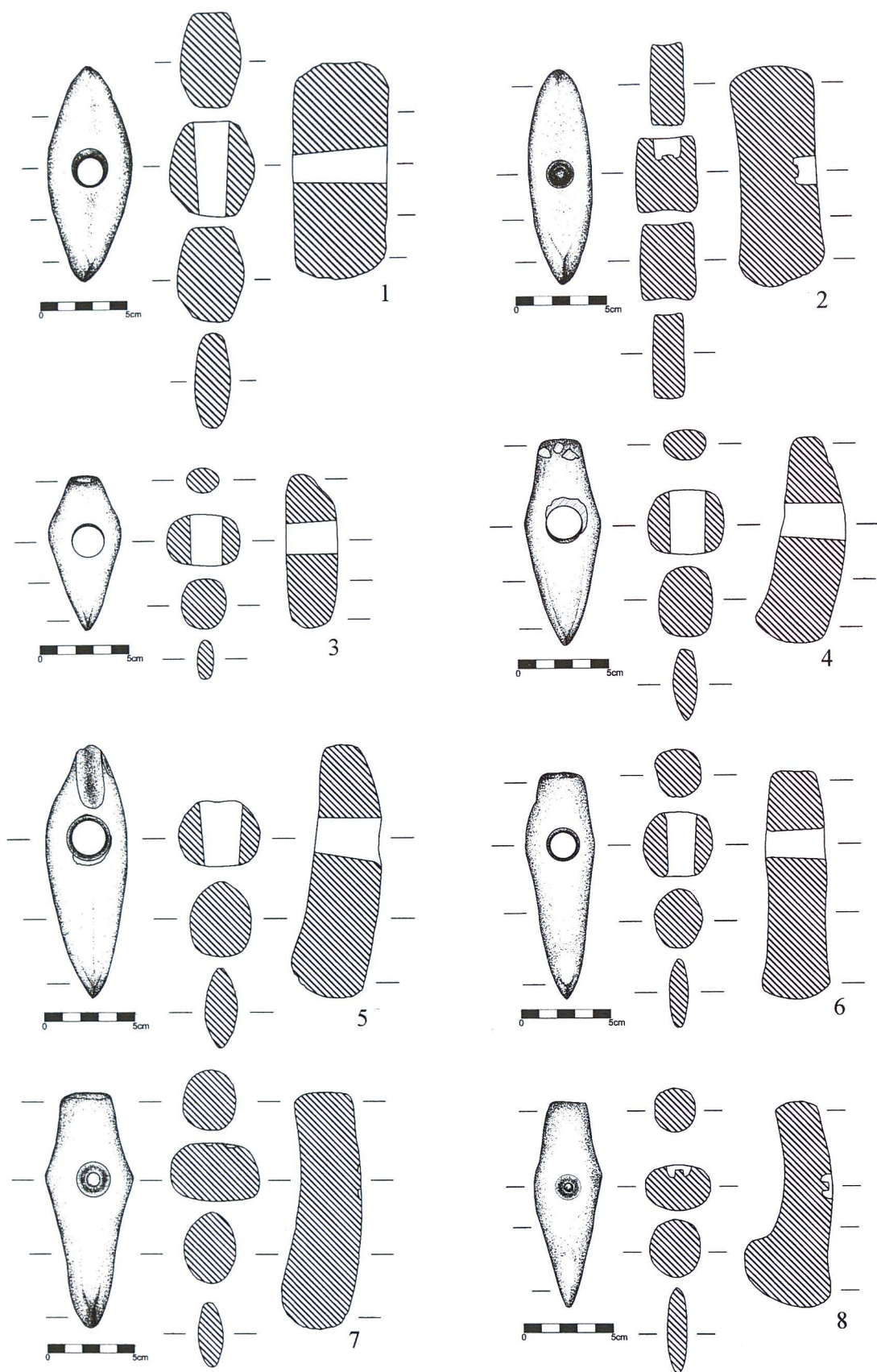
Обр. 2. Цели каменни брадви с дупка от бронзовата епоха. Случайни находки от територията на Северозападна България: 1-ИМ Белоградчик No. Бз А35; 2-РИМ Враца No. А644; 3-НАИМ-БАН No. 679; 4-НАИМ-БАН No. 644; 5-РИМ Враца No. А364; 6-НАИМ-БАН No. 3987; 7-РИМ Враца No. А292; 8-ИМ Оряхово No. 8
