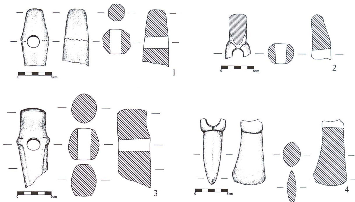
Обр. 4. Фрагменти от каменни брадви с дупка от бронзовата епоха. Случайни находки от територията на Северозападна България: 1-РИМ Враца No. A355; 2-НАИМ-БАН No. 1065; 3-РИМ Монтана No. 1168; 4-РИМ Враца No. A2993
