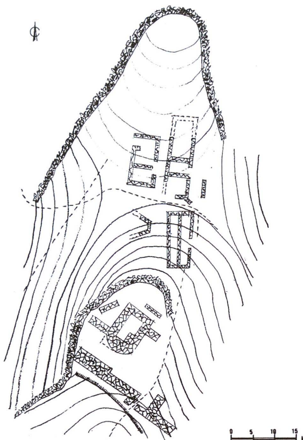
Обр. 5. Дряново. Късноантична крепост над Дряновския манастир (план В. Бараков)
