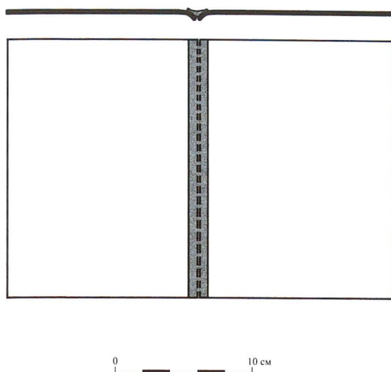
Обр. 5. Велико Търново. Техническа рисунка на начина на свързване на пластините
