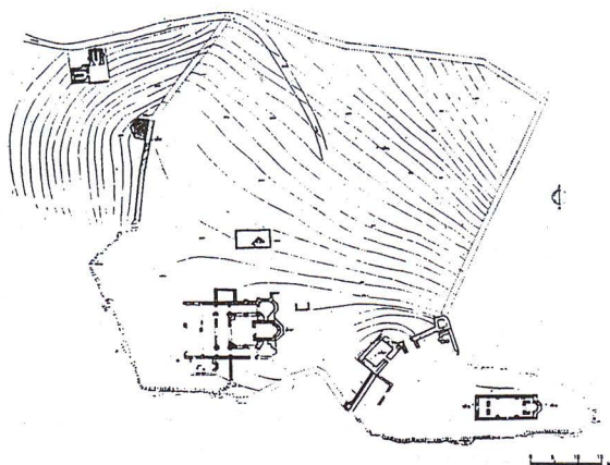
Обр. 6. Крамолин, Севлиево. Средновековна крепост от XIII-XIV в. в м. Градът (план А. Милчев, К. Койчева)
