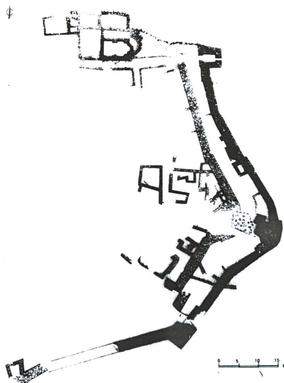
Обр. 9. Крепостта от XII-XIV в. в м. Пречиста при Градница, Севлиево (план А. Милчев)
