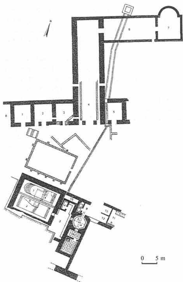
Обр. 8. Хисаря. План на късноримска баня в Диоклецианопол (по Маджаров 1993) Fig. 8. Hisariya. Plan of the late Roman baths in Diocletianopolis (after Madzharov 1993)
