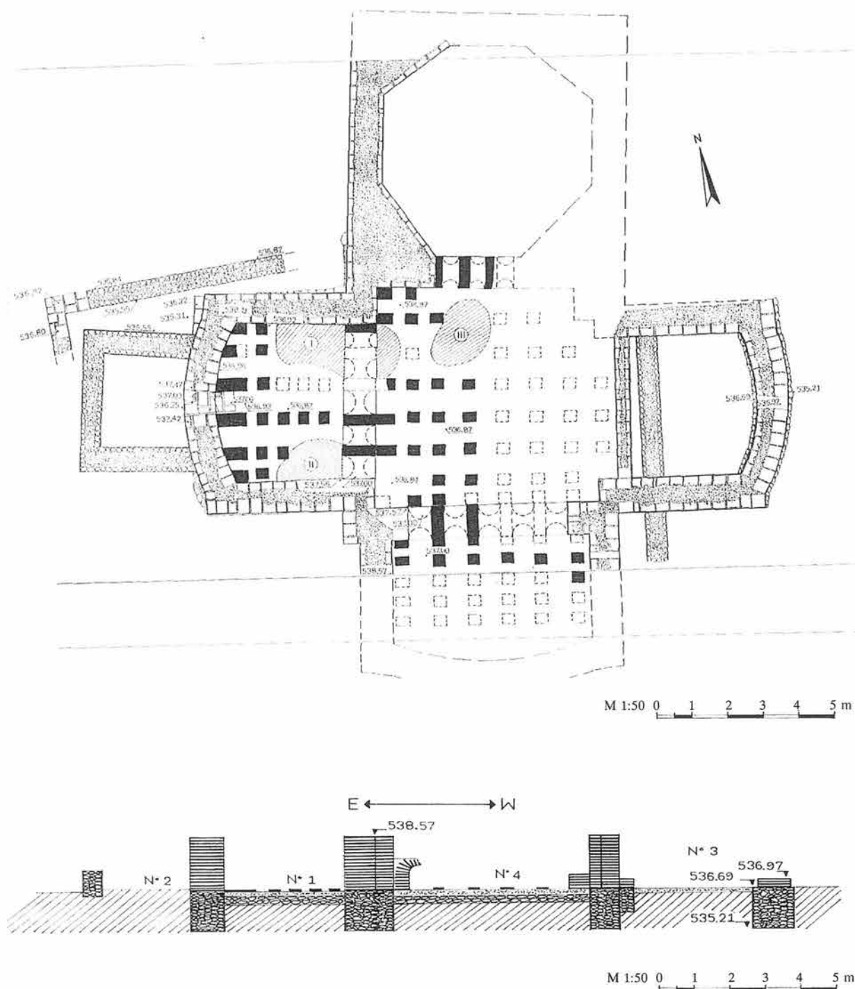
Обр. 2. Сердика. План и разрез на банята (автор К. Шалганов) Fig. 2. Serdica. Plan and section of the baths (made by K. Shalганov)
