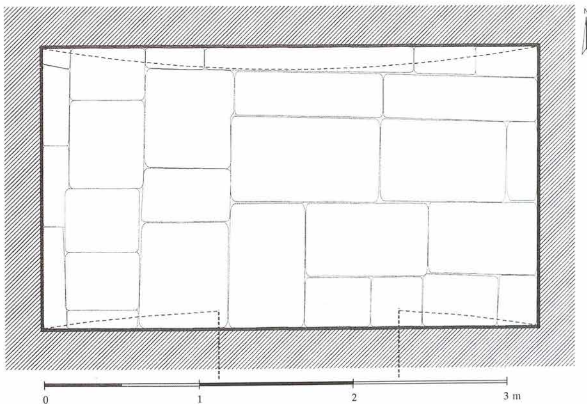
Обр. 4. Крън, Казанлъшко. Могила Светица. Саркофагоподобен гроб, план с подова настилка (Автори: архитекти Майя и Бойко Бужашки)
