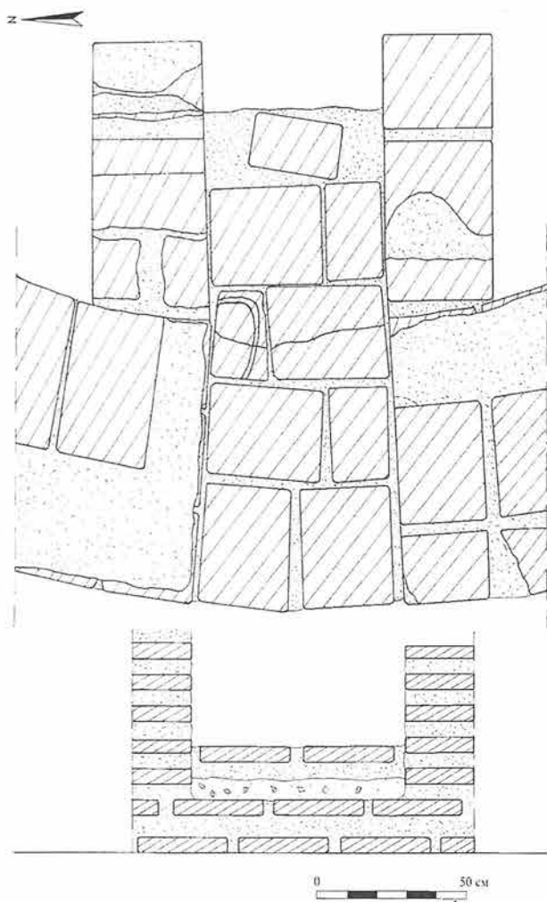
Обр. 7. Сердика. План и разрез на канала, водещ от префурниума към помещение № 1 (автор Н. Кирова) Fig. 7. Serdica. Plan and section of the connection between the praefurnium and Chamber № 1 (made by N. Kirova)
