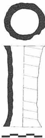
Обр. 4. Сердика. Тубули от стенно отопление Fig. 4. Serdica. Tubuli for the wall-heating
