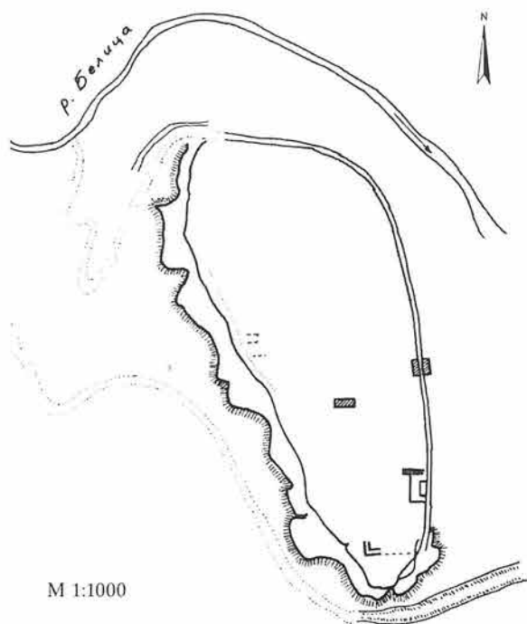
Обр. 2. Килифарево. Крепостта Градът. План (В. Бараков, Й. Алексиев) Fig. 2. Kilifarevo. Plan of the fortress at Gradat (V. Barakov, Y. Alexiev)
