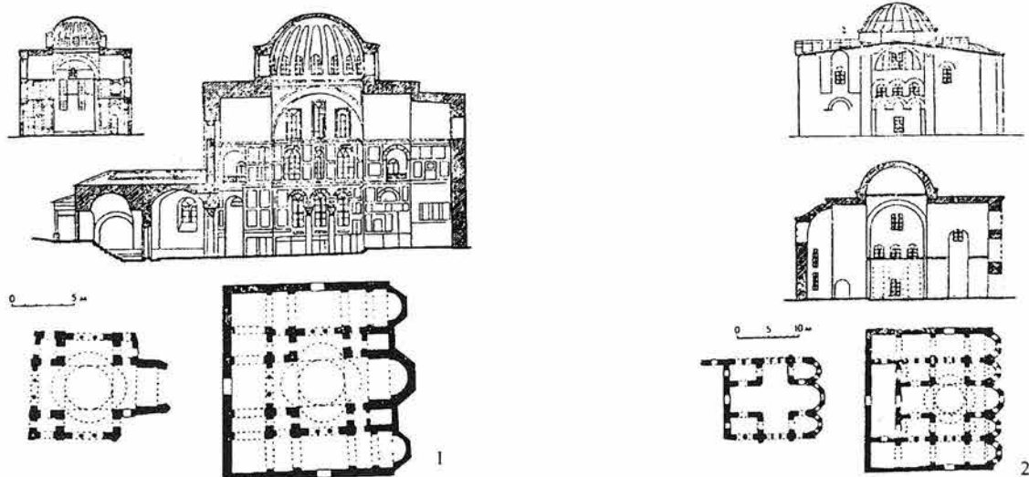
Обр. 6. Константинополски църкви от „преходен тип“: 1. Календер-джамии; 2. Атик-джамии Fig. 6. Churches of the "transition" type in Constantinople: 1 - Kalendar-cami; 2 - Atik-cami
