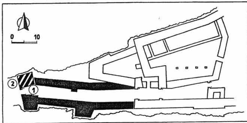
Обр. 5. Главният вход – Втори период, първи етап.
