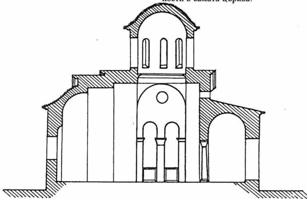
Обр. 3. Надлъжен разрез (оразмеряване и реконструкция). Fig. 3. Longitudinal Section (dimensioning and reconstruction).
