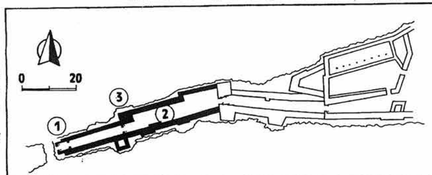
Обр. 7. Главният вход – Втори период, трети етап. 1. Четвърта порта, 2. Крепостна стълба, 3. Пета порта 7. The main entrance – The second period, third faze. 1. Forth gate, 2. Fortress staircase, 3. Fifth gate
