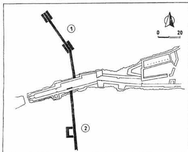
Обр. 8. Главният вход – Втори период, четвърти етап. 1. Северна напречна крепостна стена, 2. Южна напречна крепостна стена.
